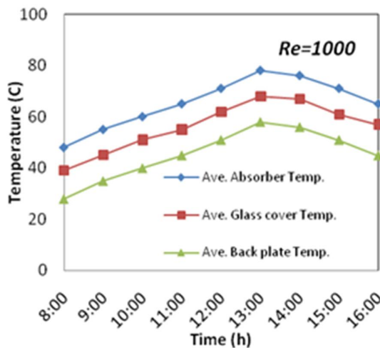
شکل ۲ دمای صفحات دستگاه بر حسب زمان (۲۱ تیرماه)
